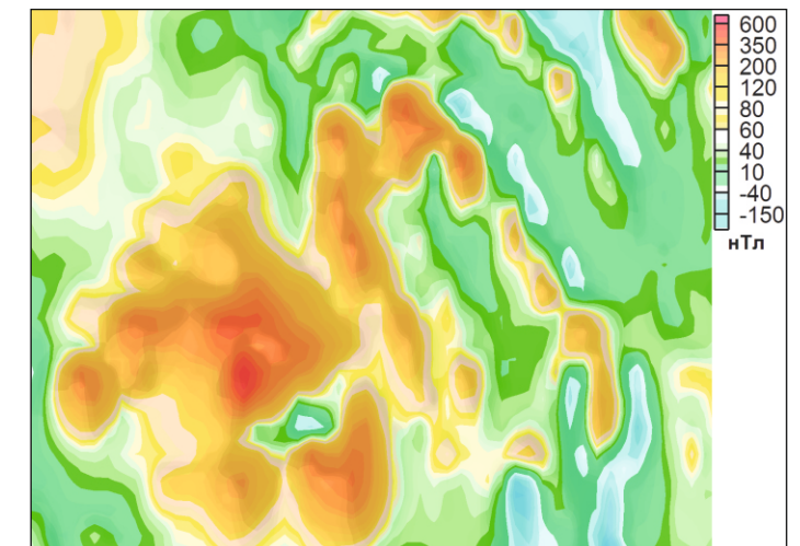
МАГНИТОМЕТРИЯ
