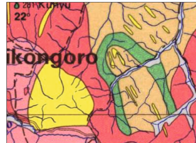
ГАММА-СПЕКТРОМЕТРИЯ
